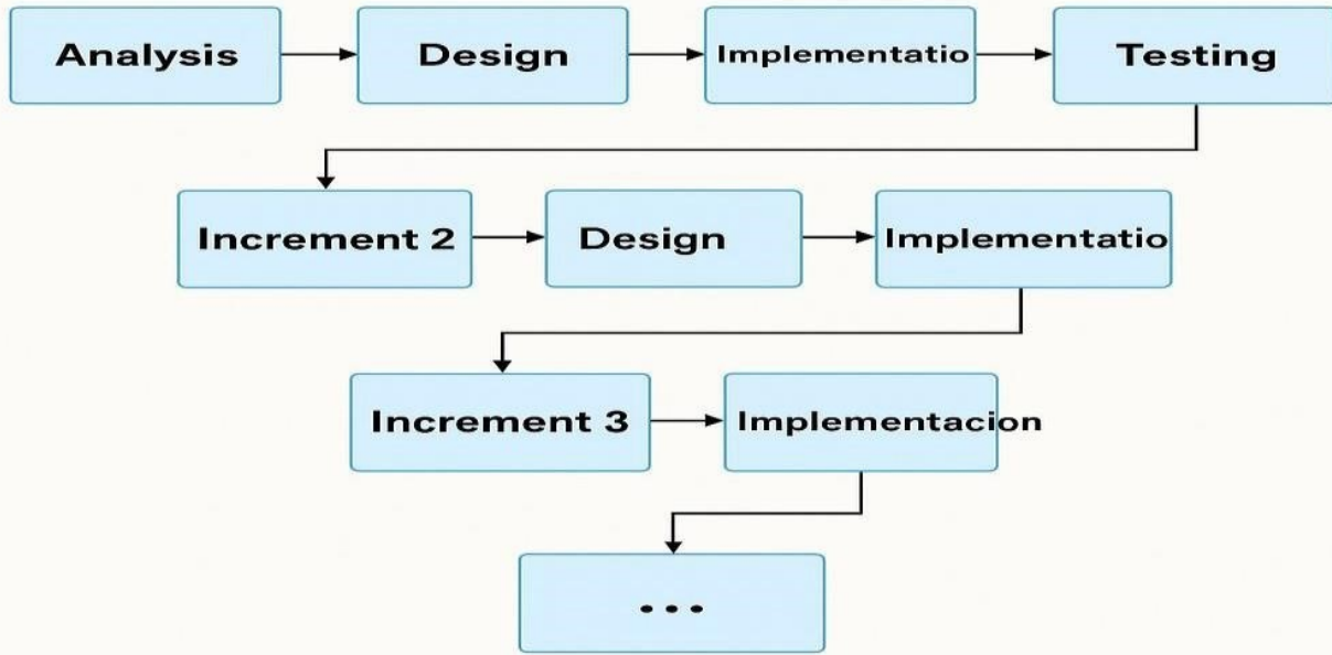
1 منهجية التطوير
