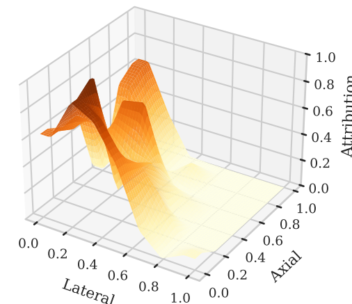
Mamba layer 1 (head)
