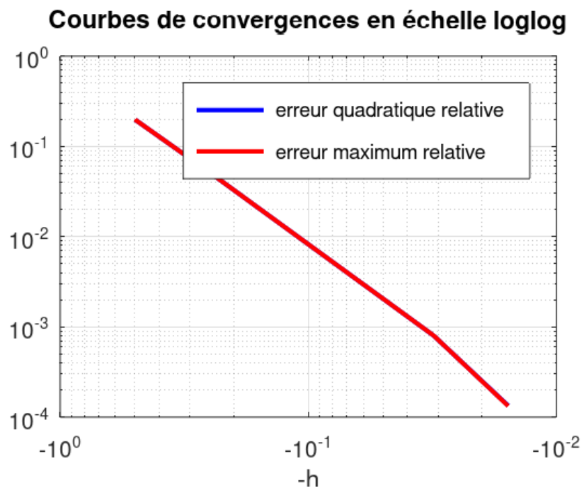
FIGURE 3 – Courbe des erreurs
