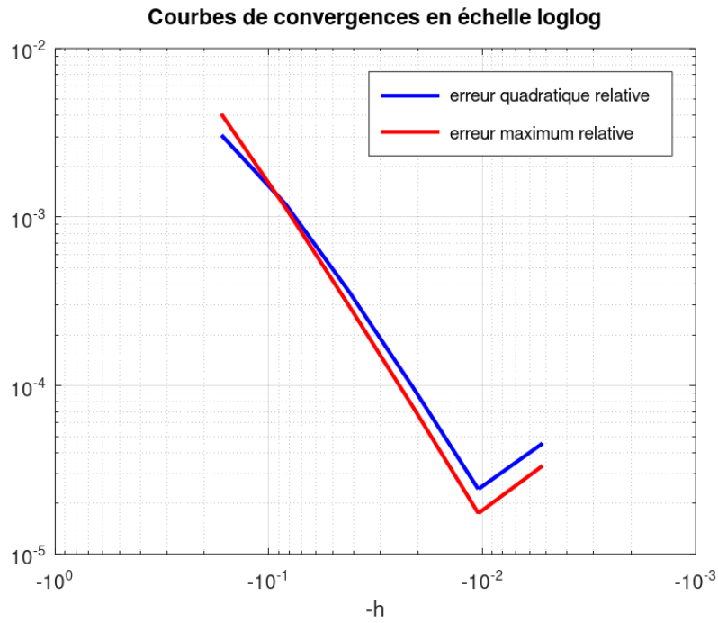
FIGURE 10 – Courbe des erreurs
