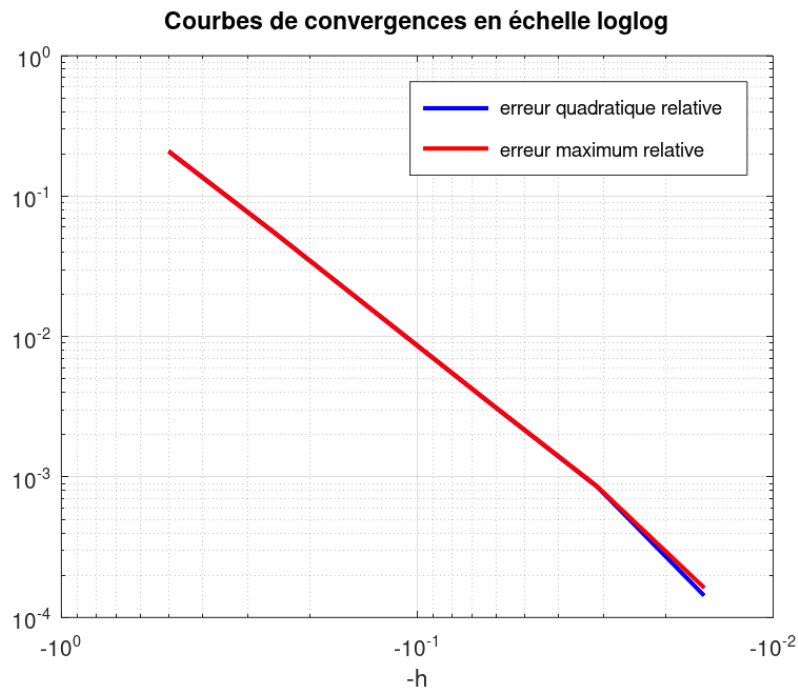
FIGURE 5 – Courbe des erreurs
