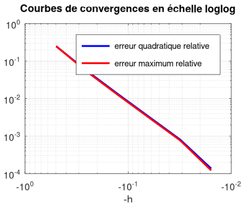
FIGURE 1 – Courbe des erreurs
