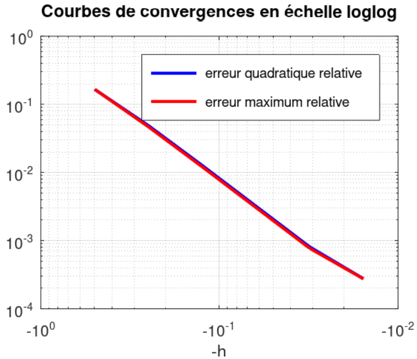
FIGURE 2 – Courbe des erreurs
