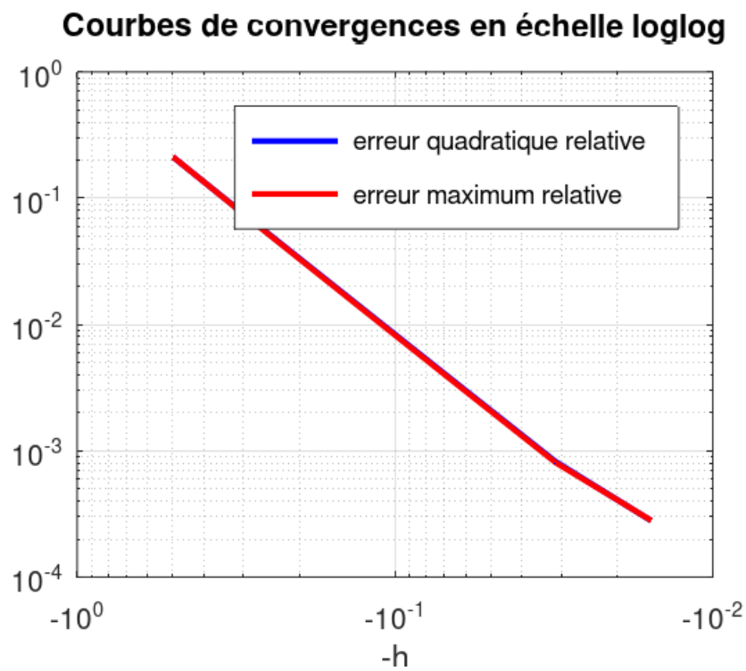
FIGURE 4 – Courbe des erreurs
