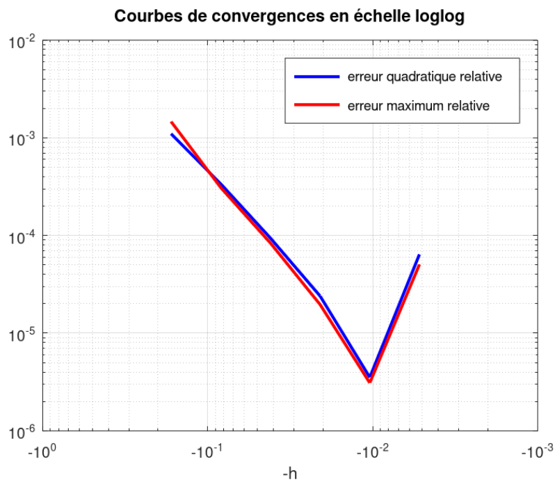
FIGURE 9 – Courbe des erreurs
