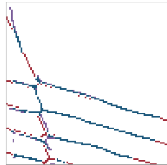
P > 0.9 F1@1 0.765
