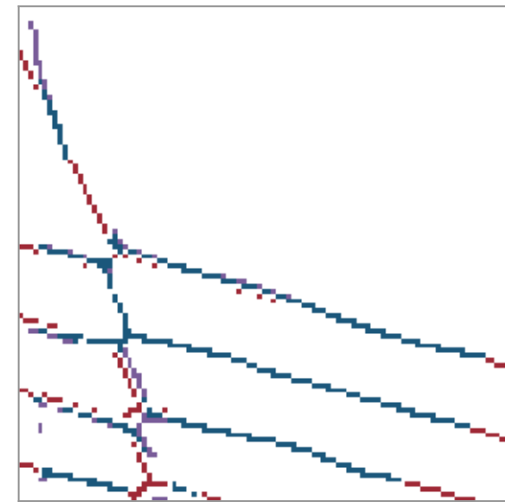
P > 0.9 F1@1 0.765
