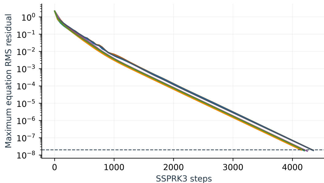
Mach 2.35
