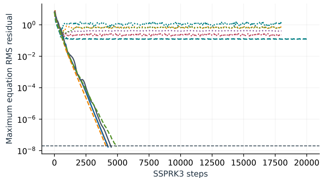
Mach 7.95
