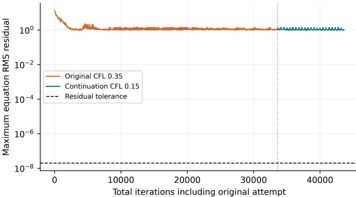
M_\infty=7.95 , N=240 : HLLC / MUSCL-MC
