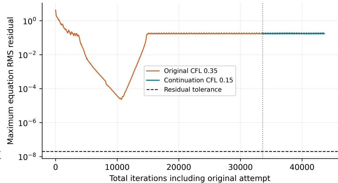
M_\infty=7.95 , N=120 : HLLC / MUSCL-MC
