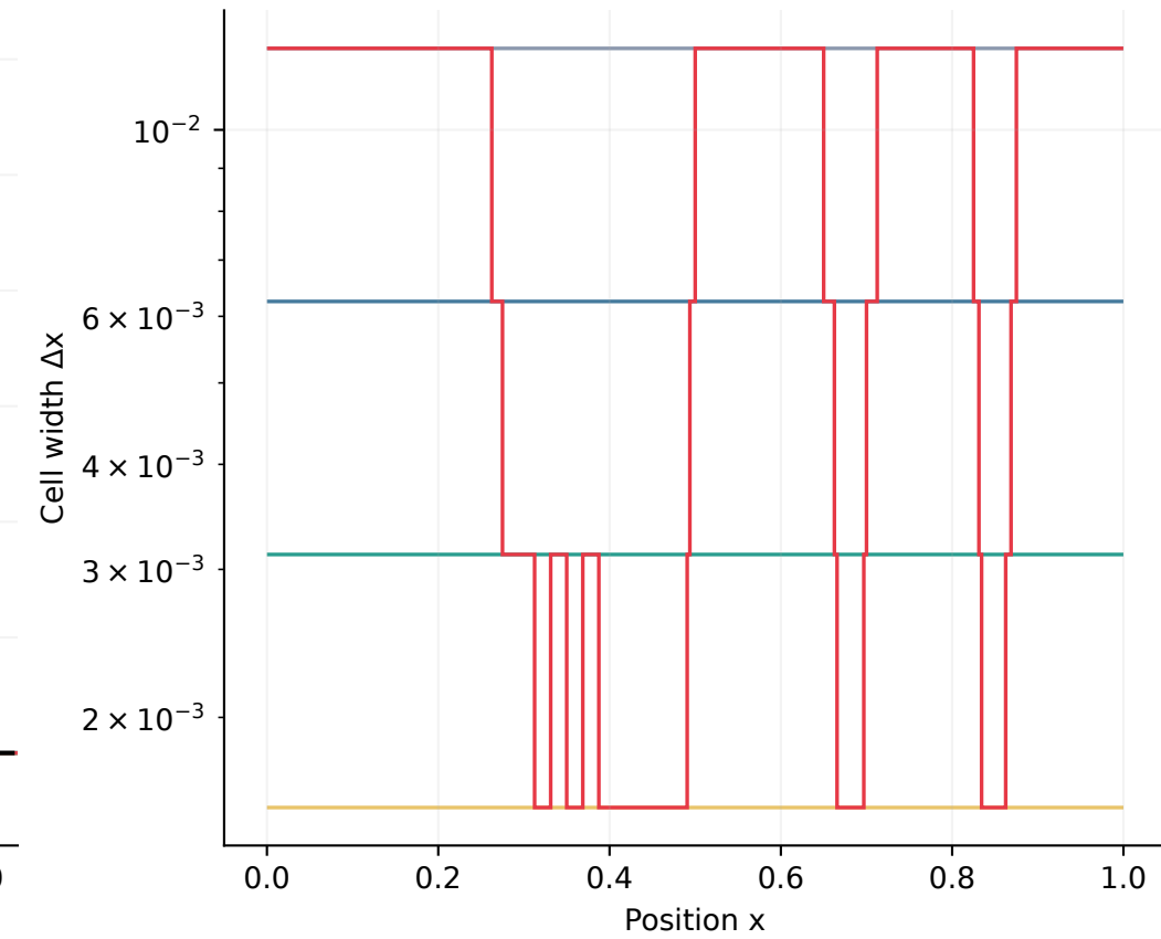
Actual final cell widths
