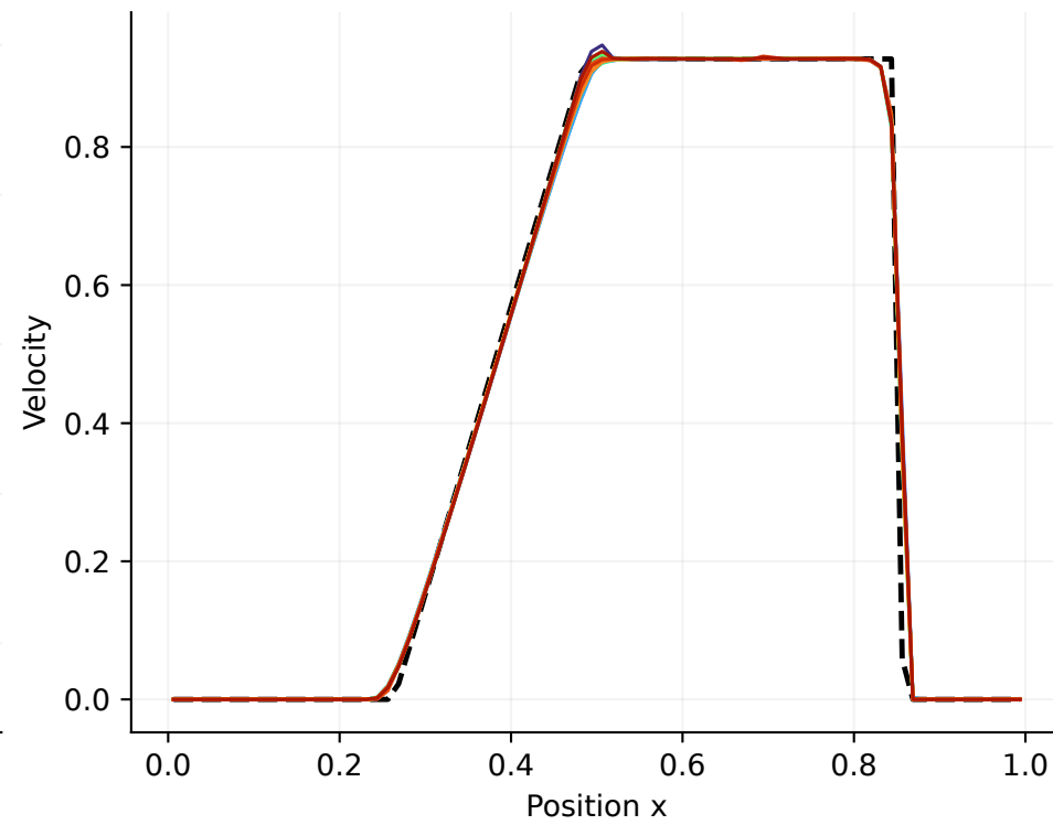
Sod · DG degree 2 · all 15 fluxes
