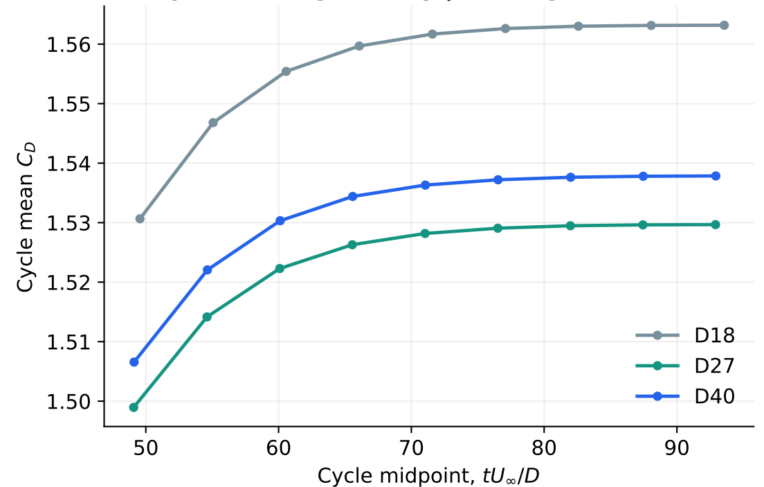
(d) Cycle-averaged drag | three grids
