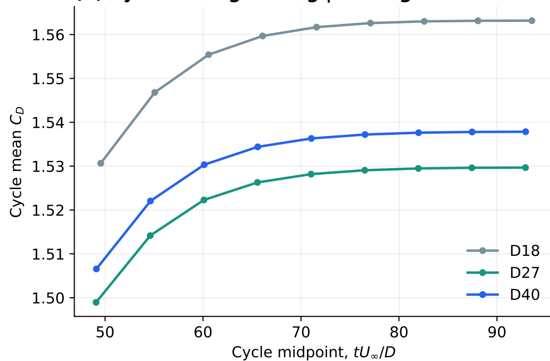
(d) Cycle-averaged drag | three grids
