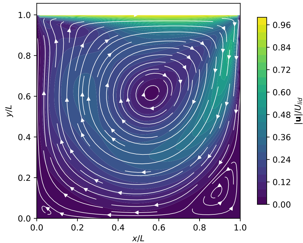
(d) CFD blind field, Re = 275
