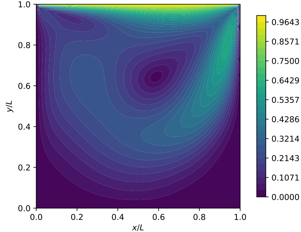
(d) CFD blind field, Re = 275
