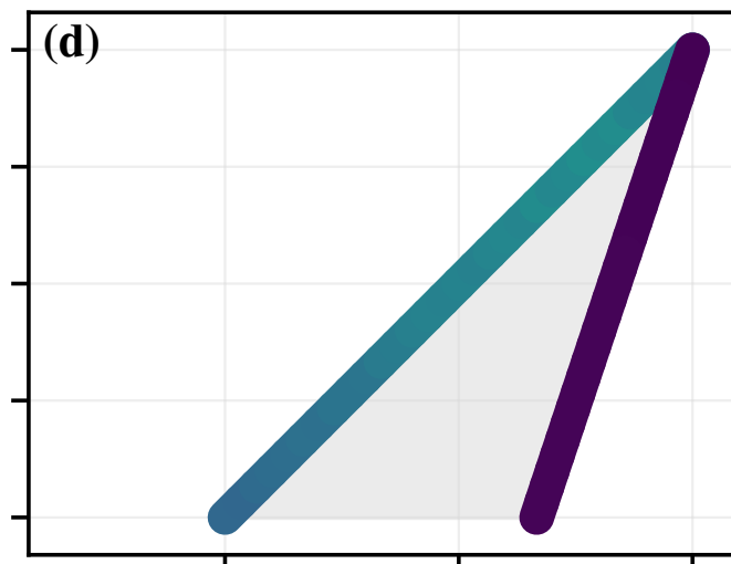
BWD, Kn=0.4 : S_{HR}
