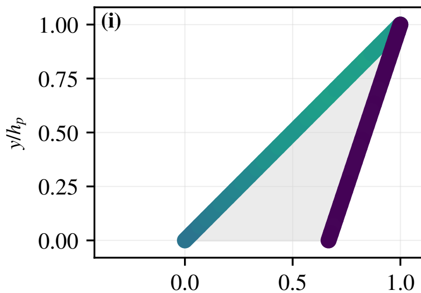
BWD, Kn=0.4 : DSMC
