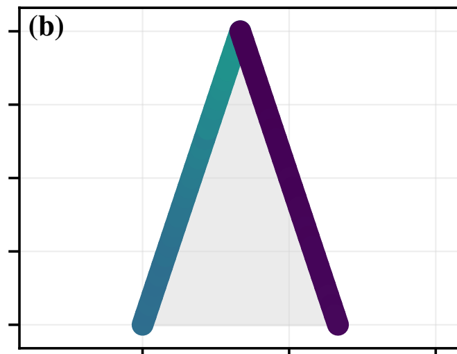
ISO, Kn=0.8 : S_{HR}
