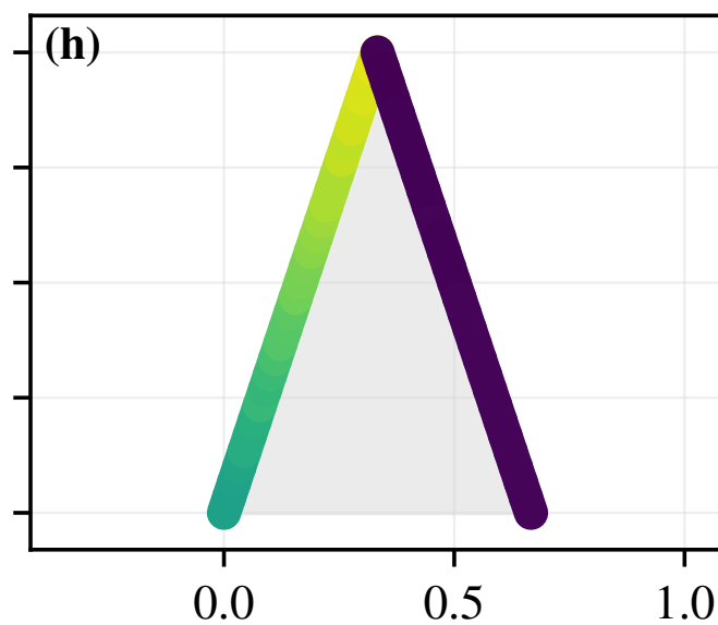
ISO, Kn=0.8 : S_{HR}
