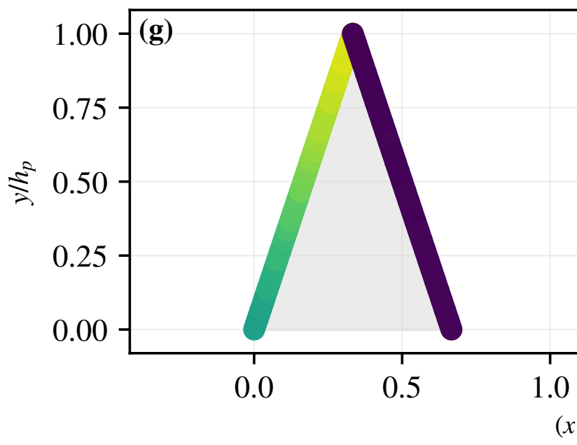
ISO, Kn=0.8 : DSMC
