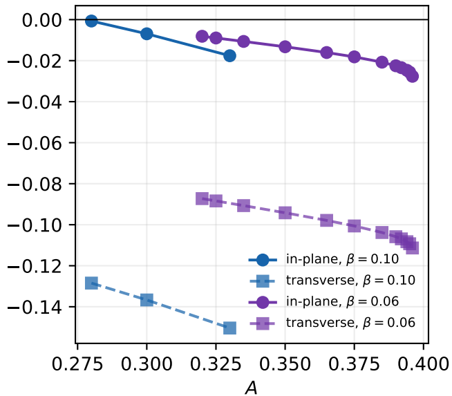
nontrivial Floquet exponent
