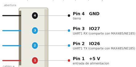
Conector 8 · MX 1.25 4P — alimentación +5 V (y UART1)
