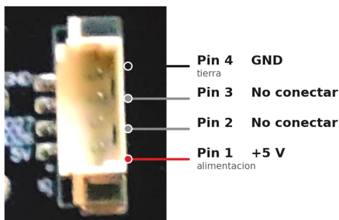
Conector 8 · MX 1.25 4P — alimentación +5 V
