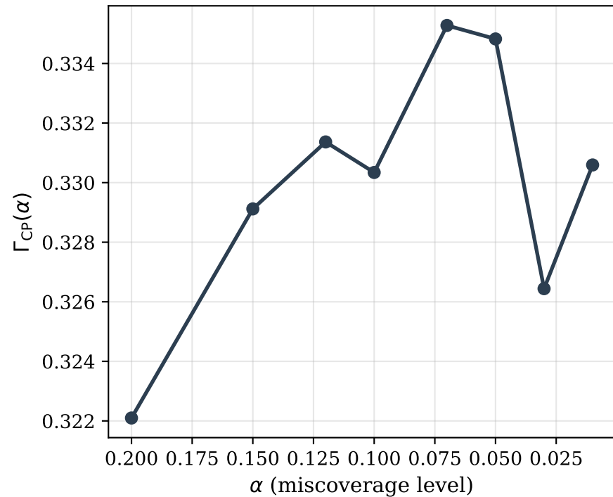
(A) Presupuesto conformal de robustez
