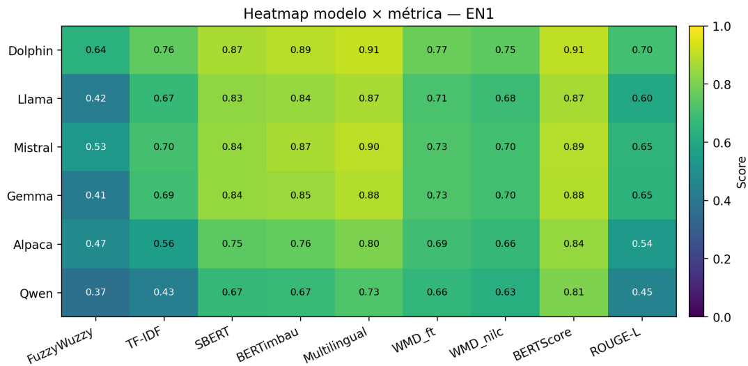
Figura 21 – Heatmap modelo × métrica em EN1.
