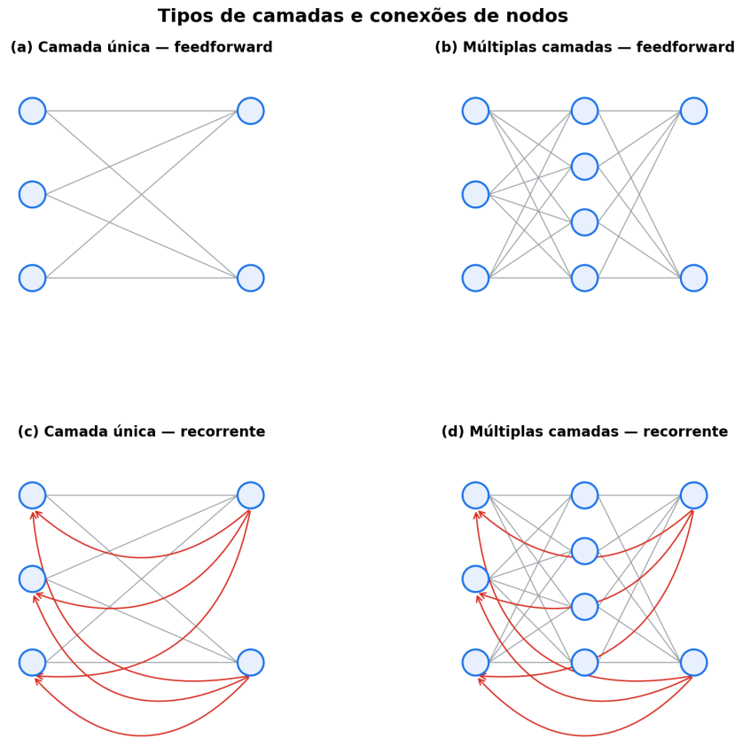
Figura 8 – Tipos de camadas e conexões de nodos.
