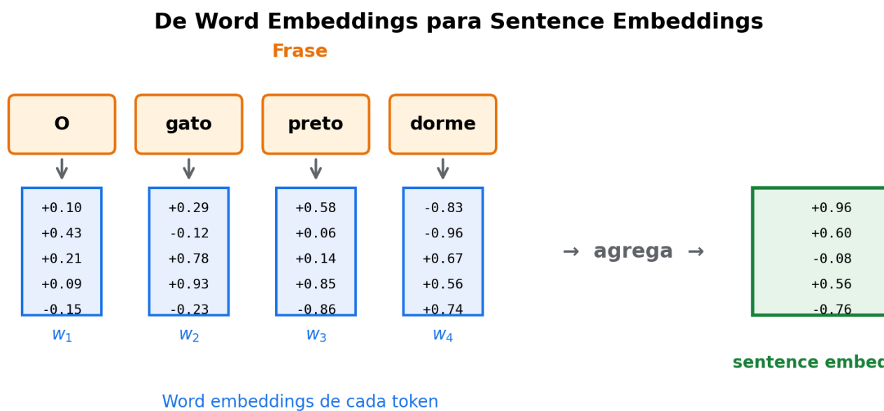
Figura 4 – Exemplo da transformação de word embeddings para sentence embeddings .
