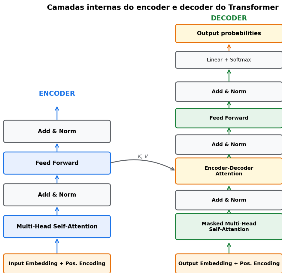
Figura 13 – Camadas do encoder e decoder do transformer .
