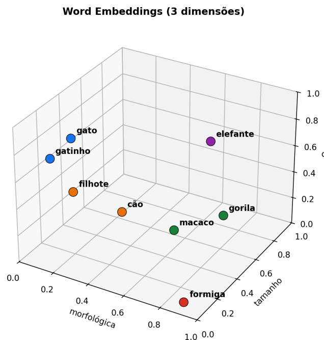
Figura 3 – Exemplo da transformação de palavras em word embeddings .
