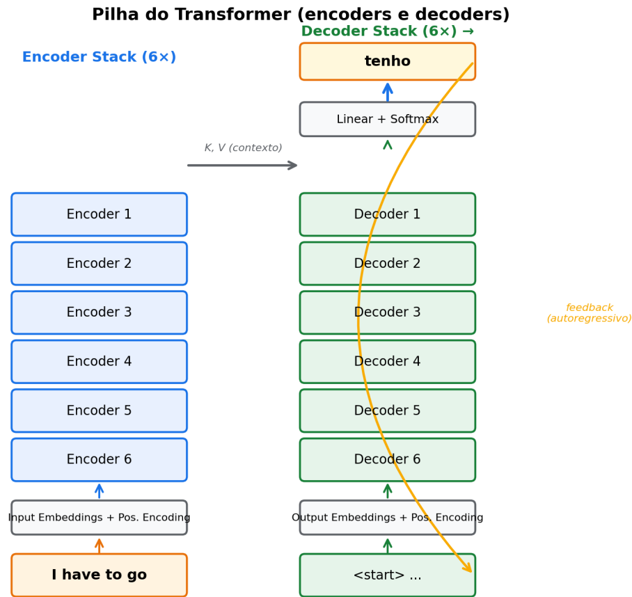
Figura 12 – Representação da pilha ( stack ) do transformer .
