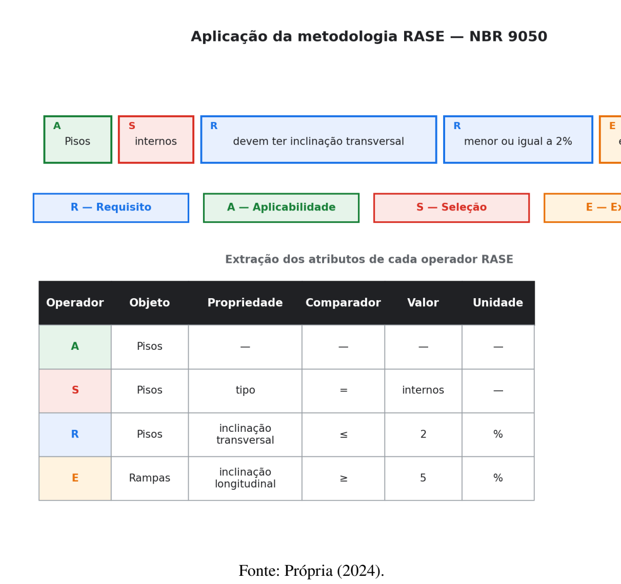
Figura 14 – Utilização da metodologia RASE na NBR 9050
