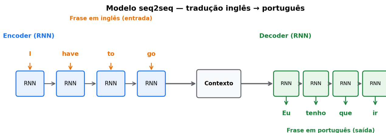
Figura 9 – Exemplo de um modelo seq2seq para tradução do inglês para português.
