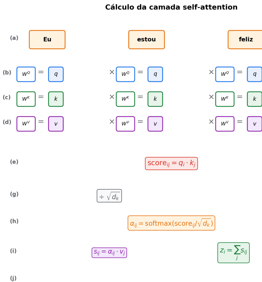
Figura 11 – Exemplo do cálculo de uma camada de self-attention .
