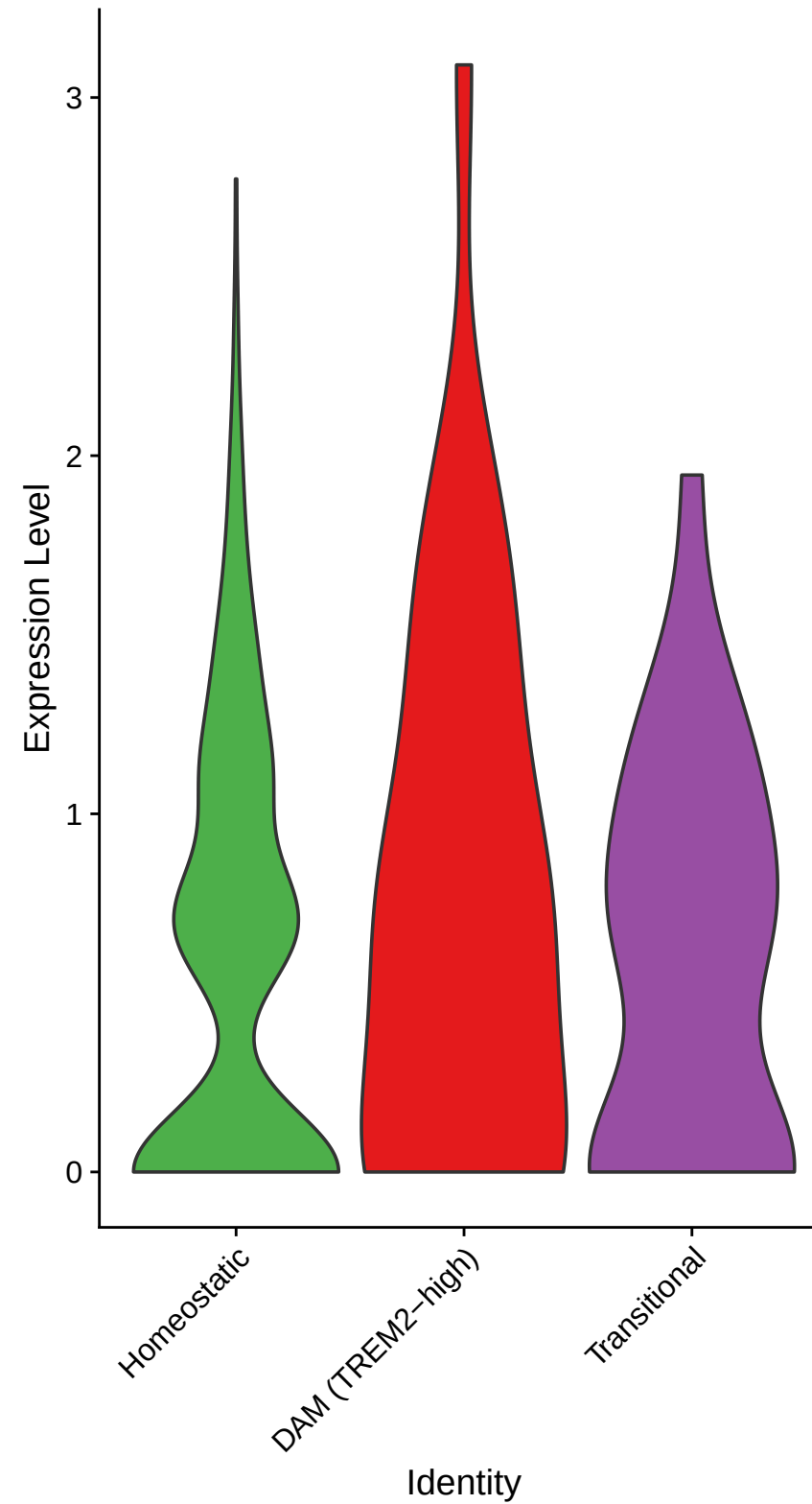
APOE
