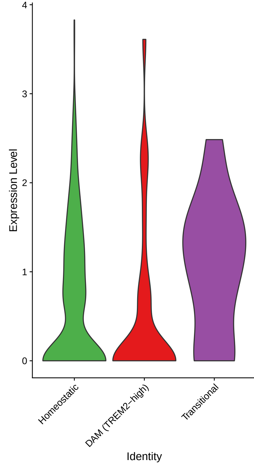
SPP1
