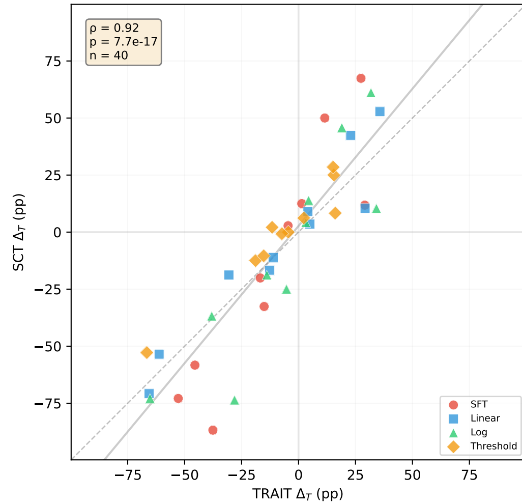
TRAIT vs SCT
