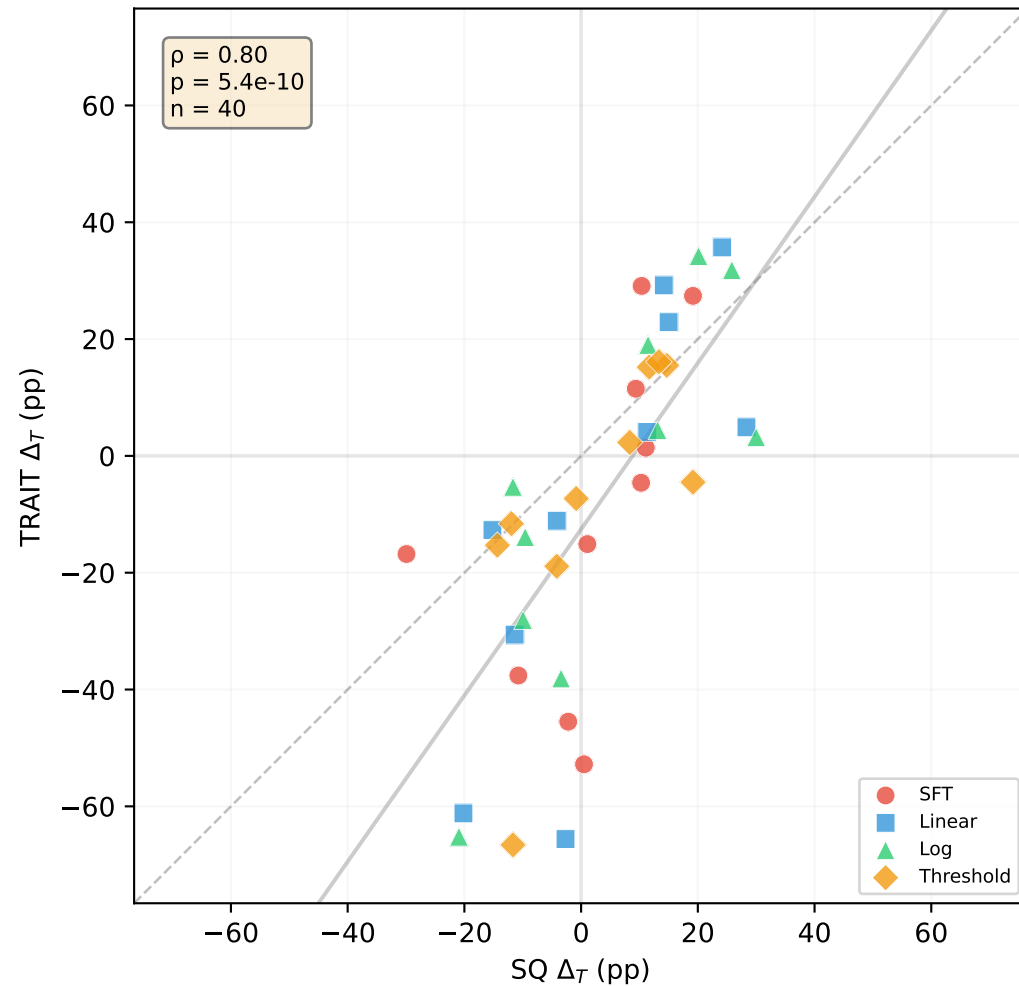
SQ vs TRAIT
