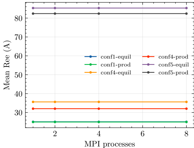
Ree vs np
