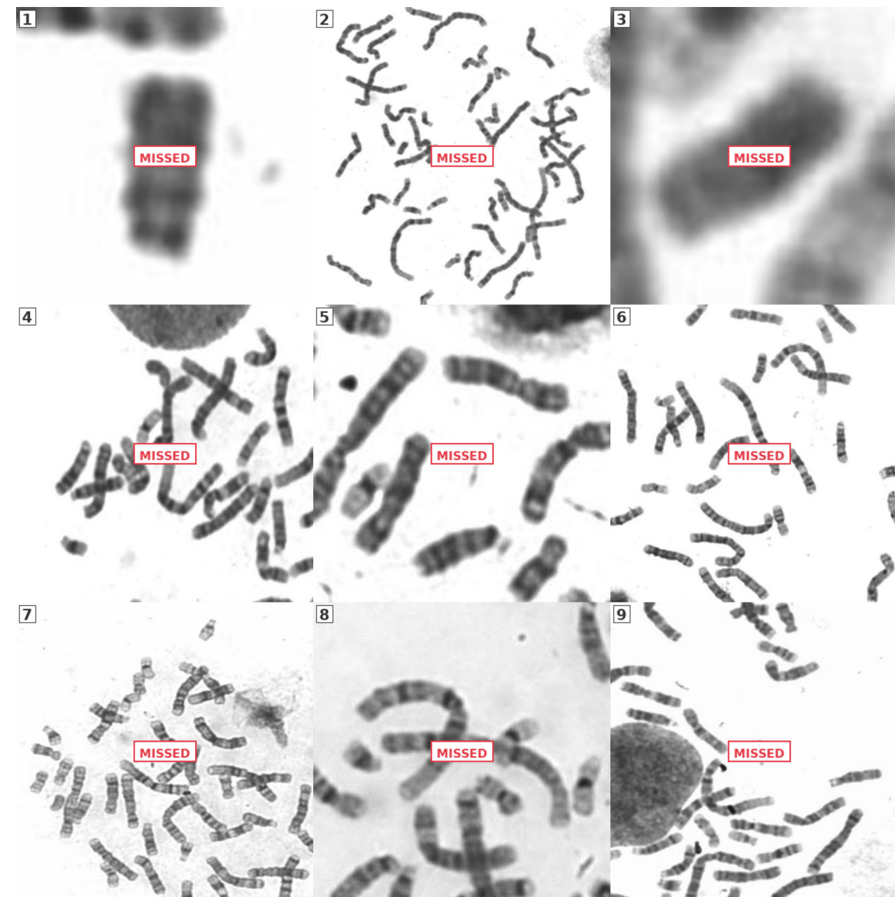
Baseline (DiffusionDet)
