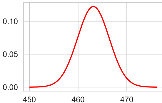
Posterior Probability Distributions
