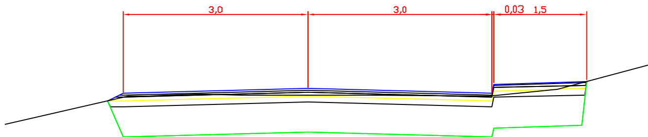
Fig: Typisk snitt Lekvebakken
