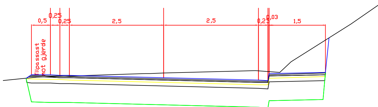
Fig: Typisk snitt Gullfjordungveg
