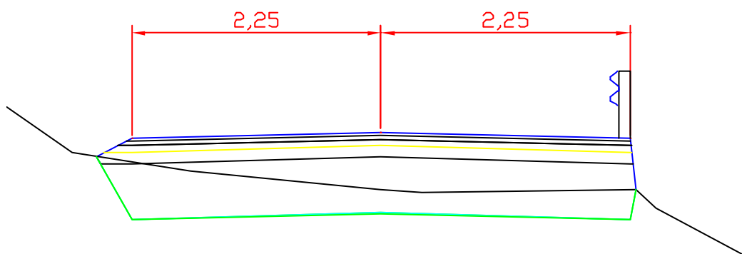
Fig: Typisk snitt Lekvebakken
