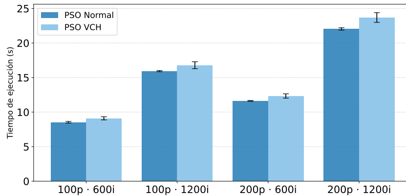
Figura 6.18: Tiempos de ejecución de Nobel. Intervalos de confianza al 95 % Fuente: Elaboración propia.
