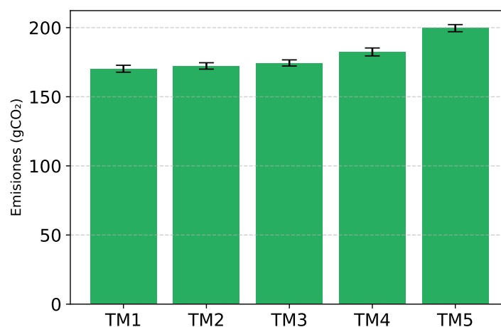
Figura 6.16: Emisiones de Nobel tras ejecutar PSO VCH 20 veces por TM con 200 partículas y 1200 iteraciones. Intervalos de confianza al 95 %
