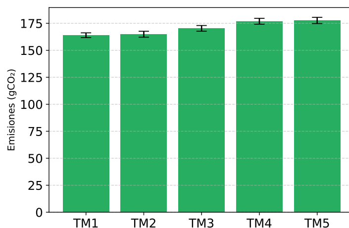
Figura 6.15: Emisiones de Geant tras ejecutar PSO VCH 20 veces por TM con 200 partículas y 1200 iteraciones. Intervalos de confianza al 95 %
