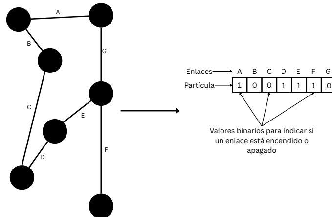
Figura 5.3: Representación de una red sencilla como partícula de pso.
