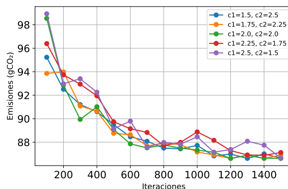
(b) Barrido con partículas fijas en 200. Fuente: Elaboración propia.
