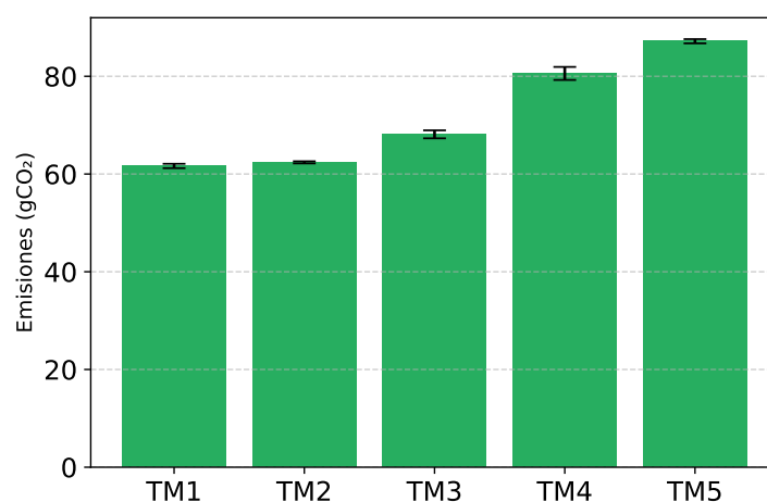
Figura 6.6: Emisiones de Abilene tras ejecutar PSO VCH 20 veces por TM con 200 patículas y 1200 iteraciones. Intervalos de confianza al 95 %
