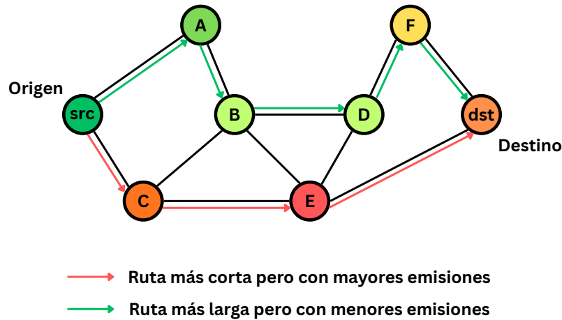
Figura 1.2: Representación gráfica del enrutamiento del tráfico a través de caminos de bajas emisiones.
