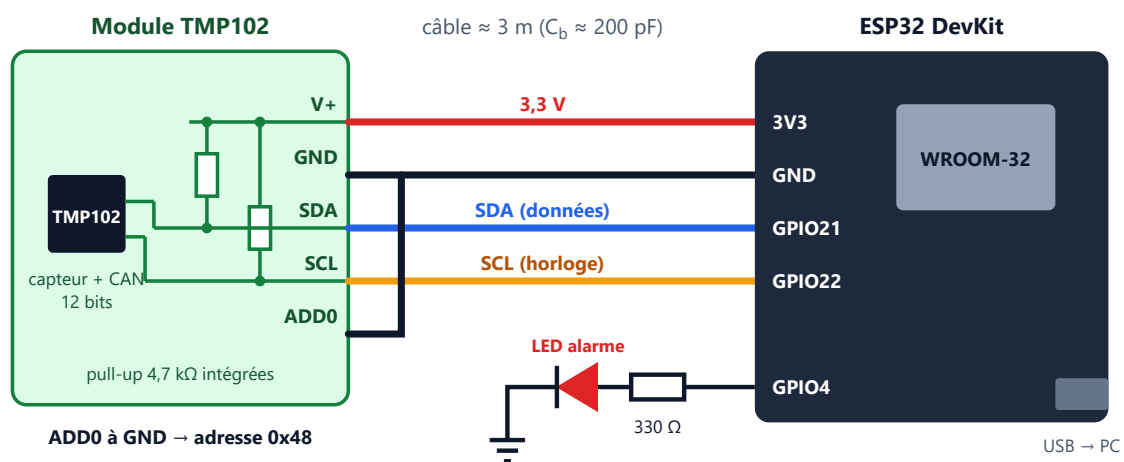
Figure 1 — Synoptique du module de supervision
