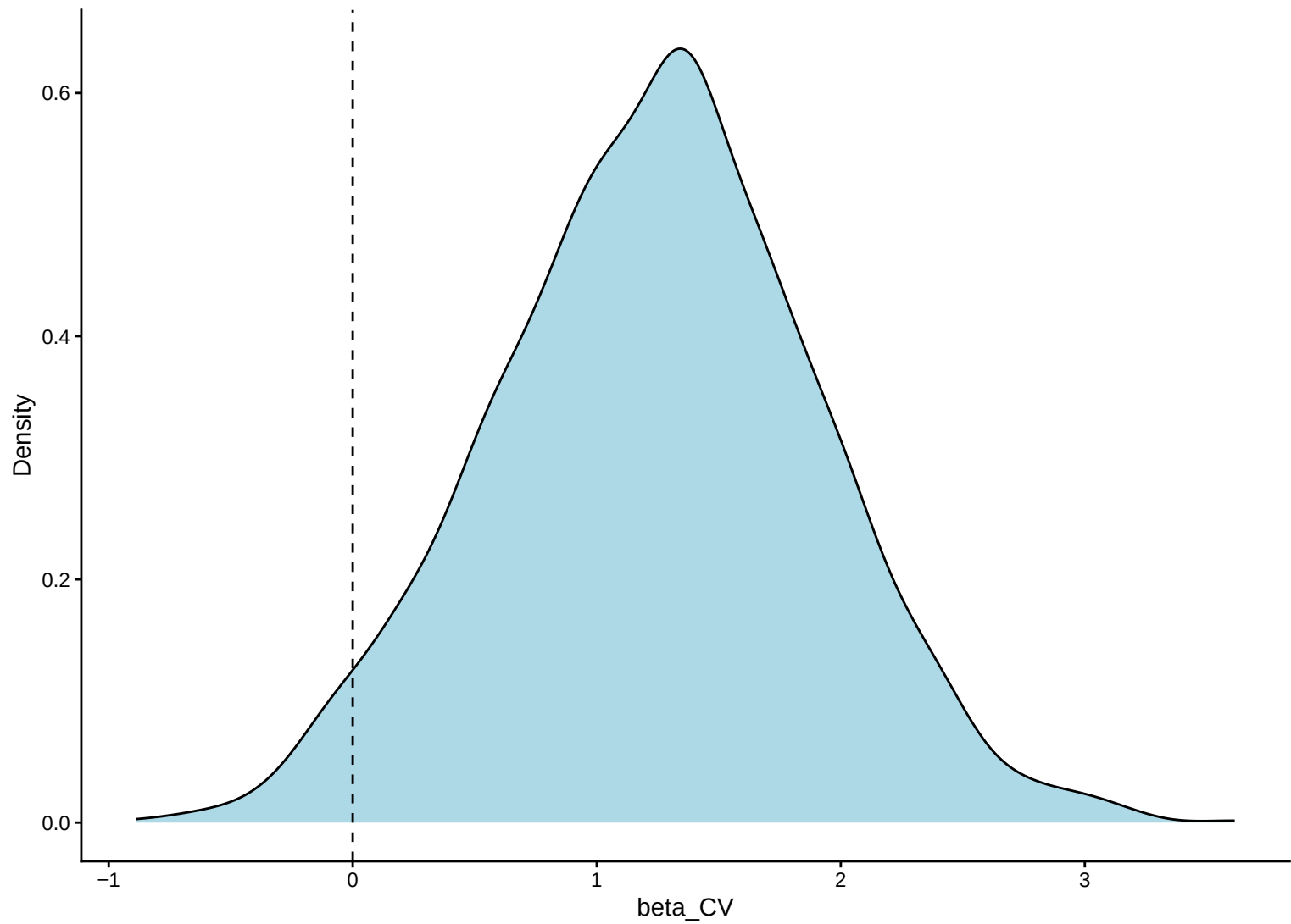
Posterior distribution of \beta_{CV}
