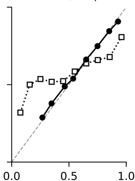
EdNet-KT1, simpleKT
