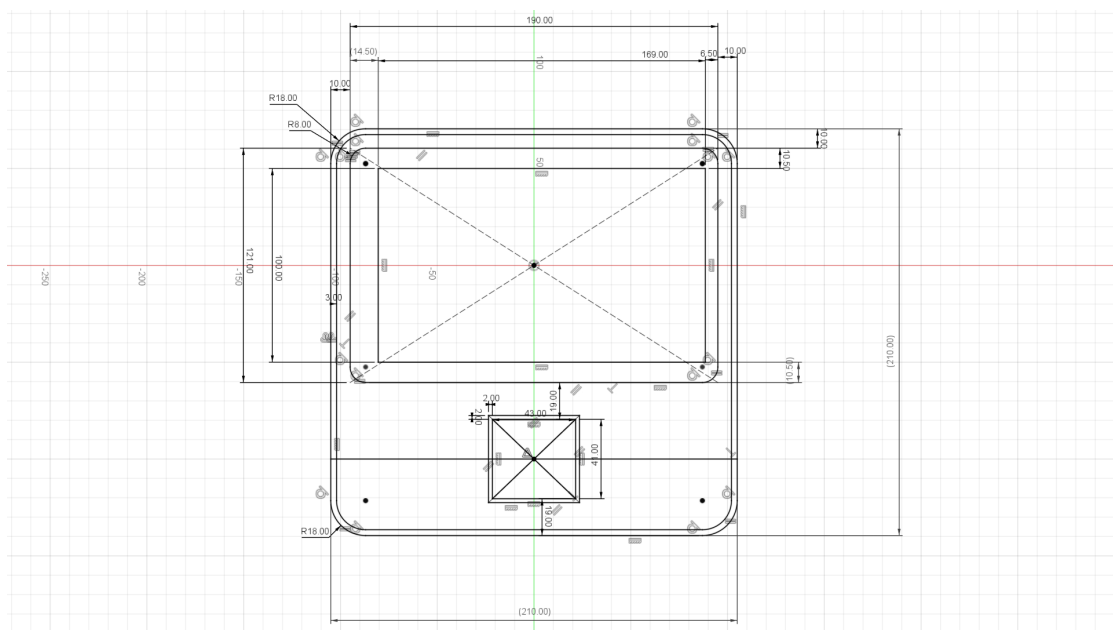
Rysunek 7.18: Rysunek techniczny panelu przedniego modułu sprzętowego.
