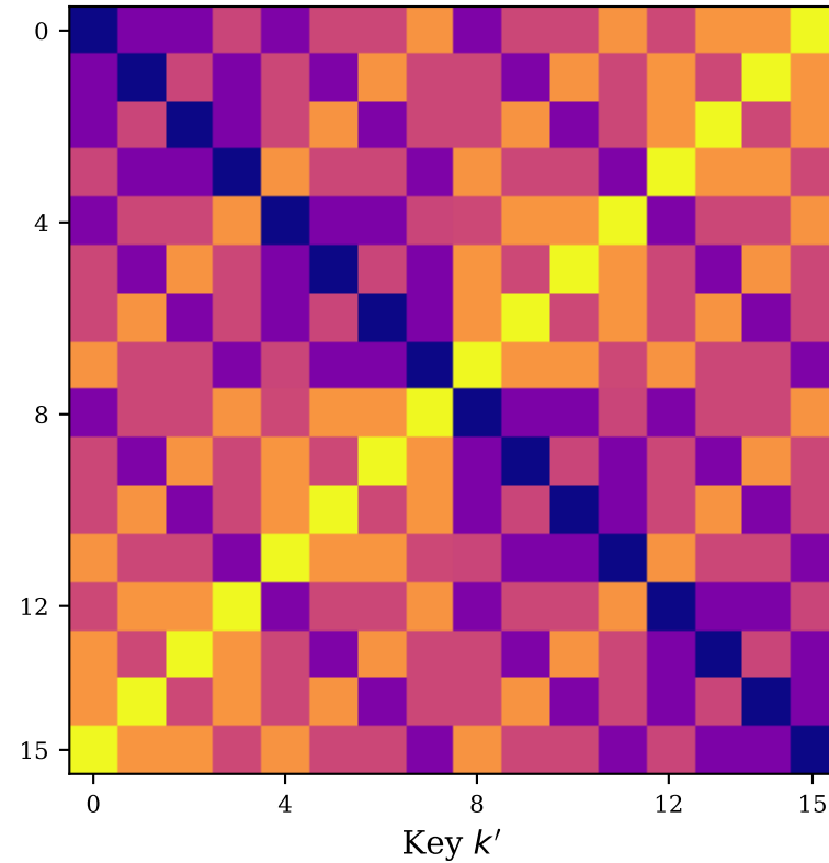
GIFT
