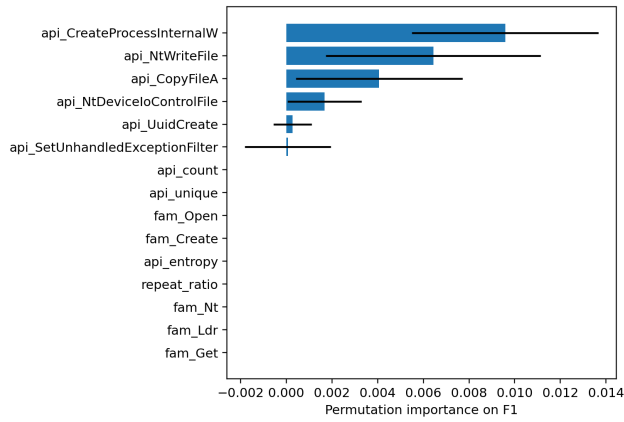
Fig. S2. Held-out permutation importance on MalBehavD-V1.
