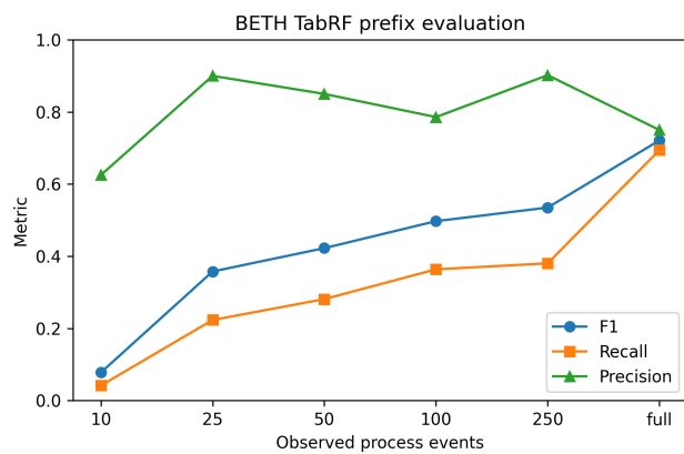
Fig. S4. BETH TabRF prefix evaluation.
