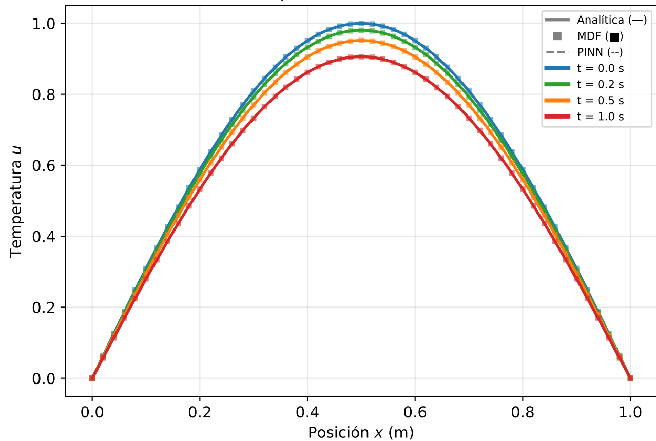
Perfiles de temperatura: Analítica vs MDF vs PINN
