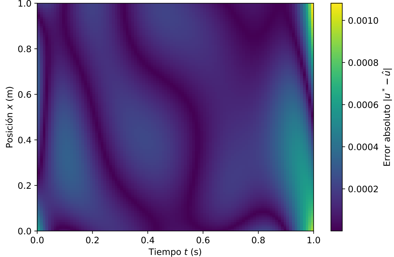
Error absoluto PINN sobre el dominio (x, t)
