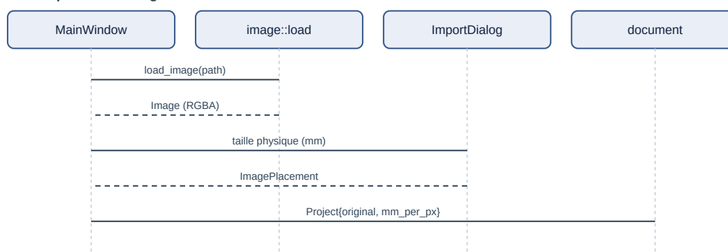
Séquence — import d'une image
