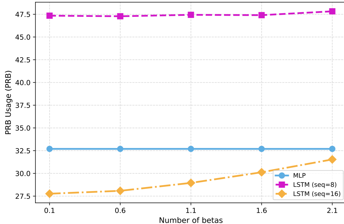
PRB Usage (PRB) - eMBB
