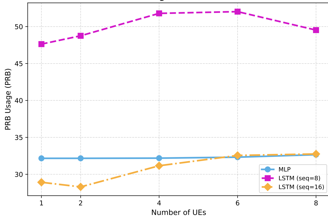
PRB Usage (PRB) - eMBB
