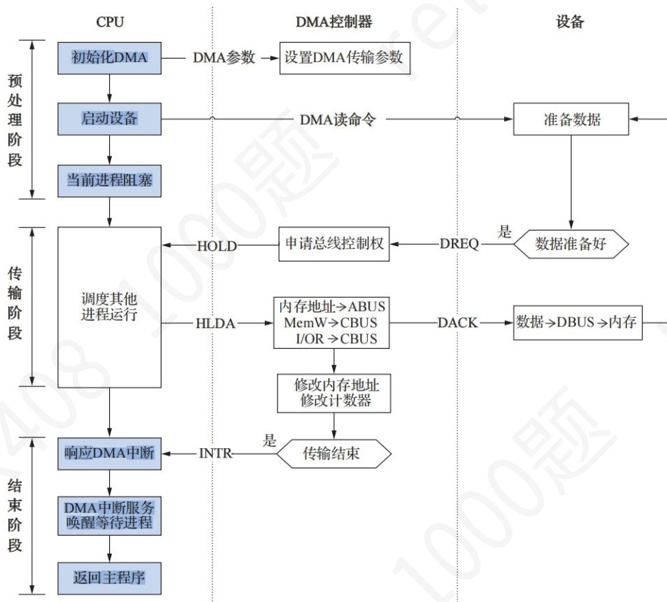
图 9.23 DMA 读操作详细流程（周期挪用）
