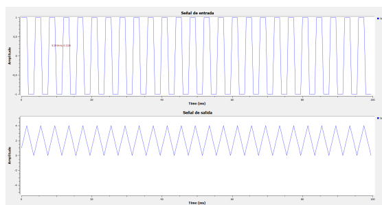
Figura 4: Señal de entrada y salida del acumulador con frecuencia de muestreo de 2 kHz.
