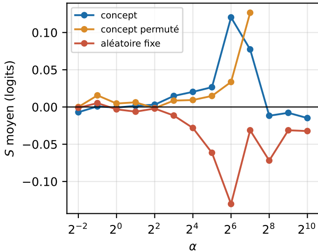
Bloc 32 : le signe sépare les familles
