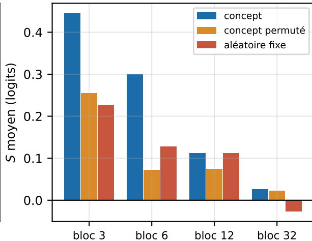
Le contrôle par permutation
