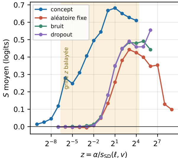
standardisation par s_{SD}
