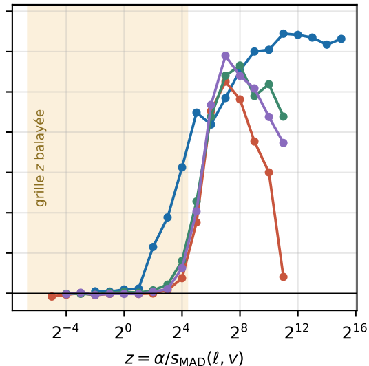
standardisation par s_{MAD}
