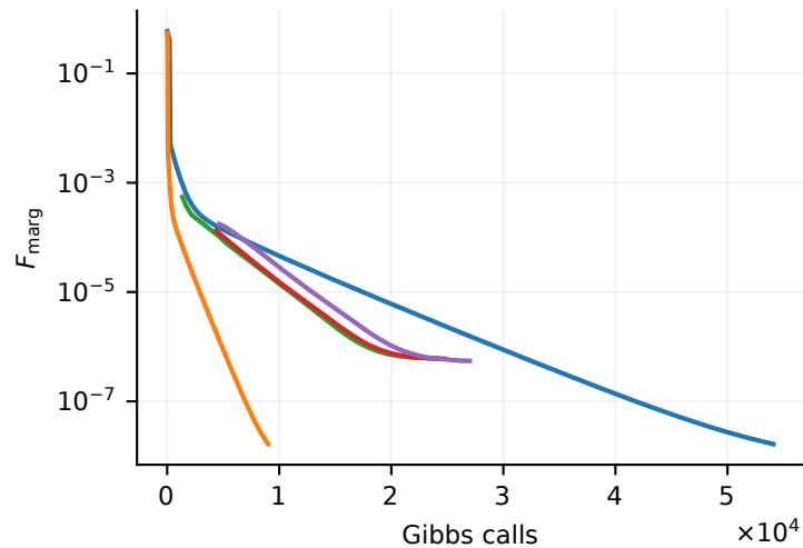
(b) Marginal KL error
