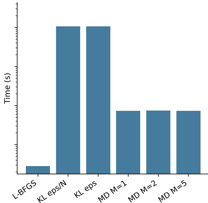
Wasserstein WP, d=20
