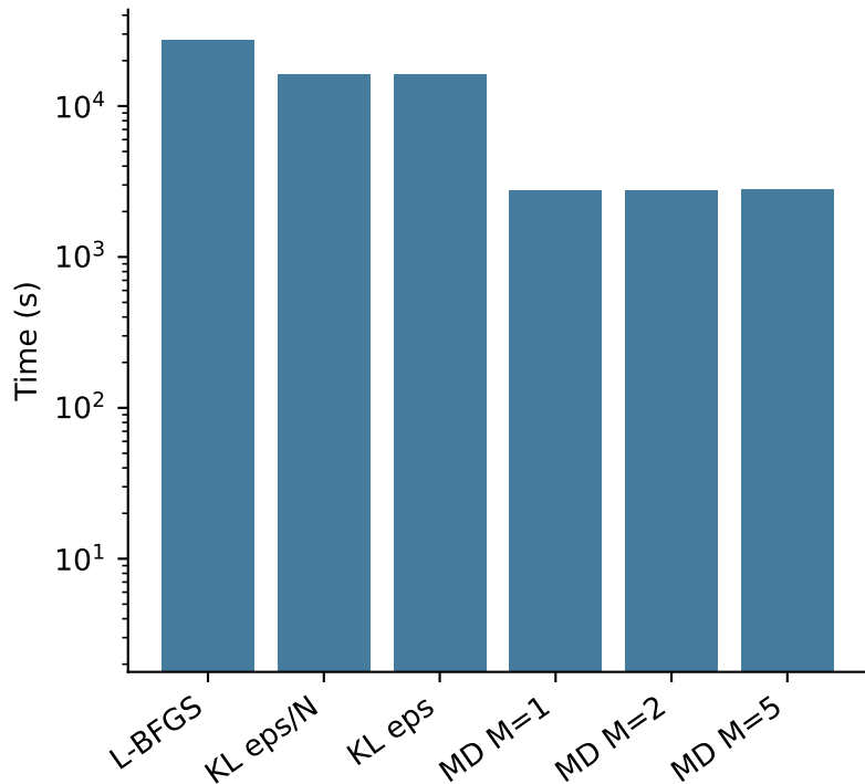
Wasserstein WC, d=20
