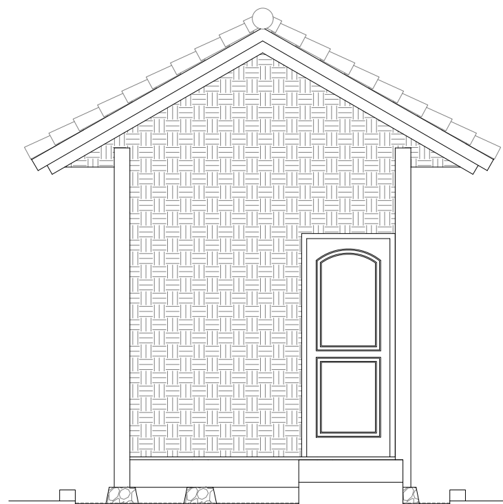
TAMPAK DEPAN SKALA 1:50
