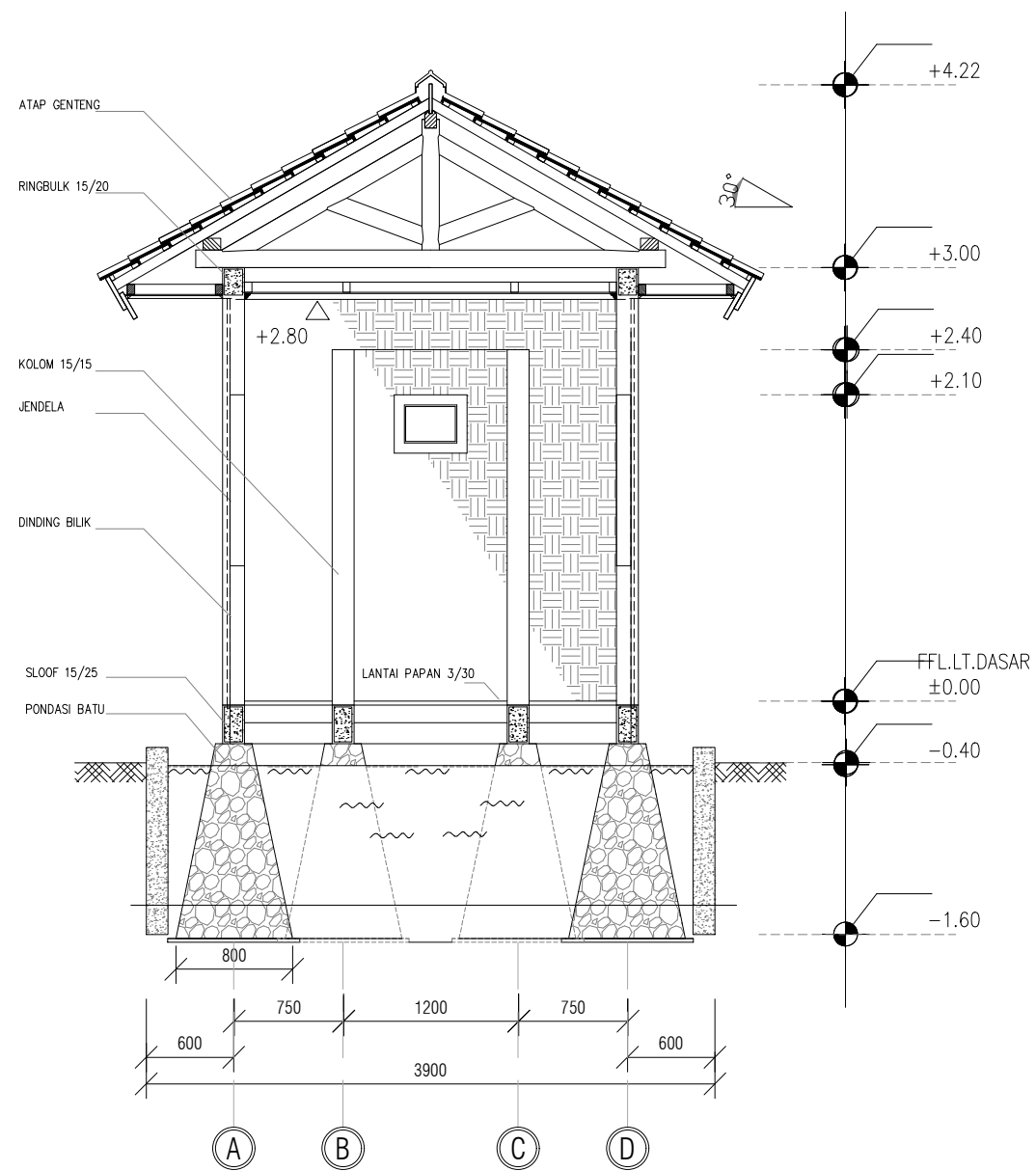
ARS POTONGAN A-A SKALA 1:50
