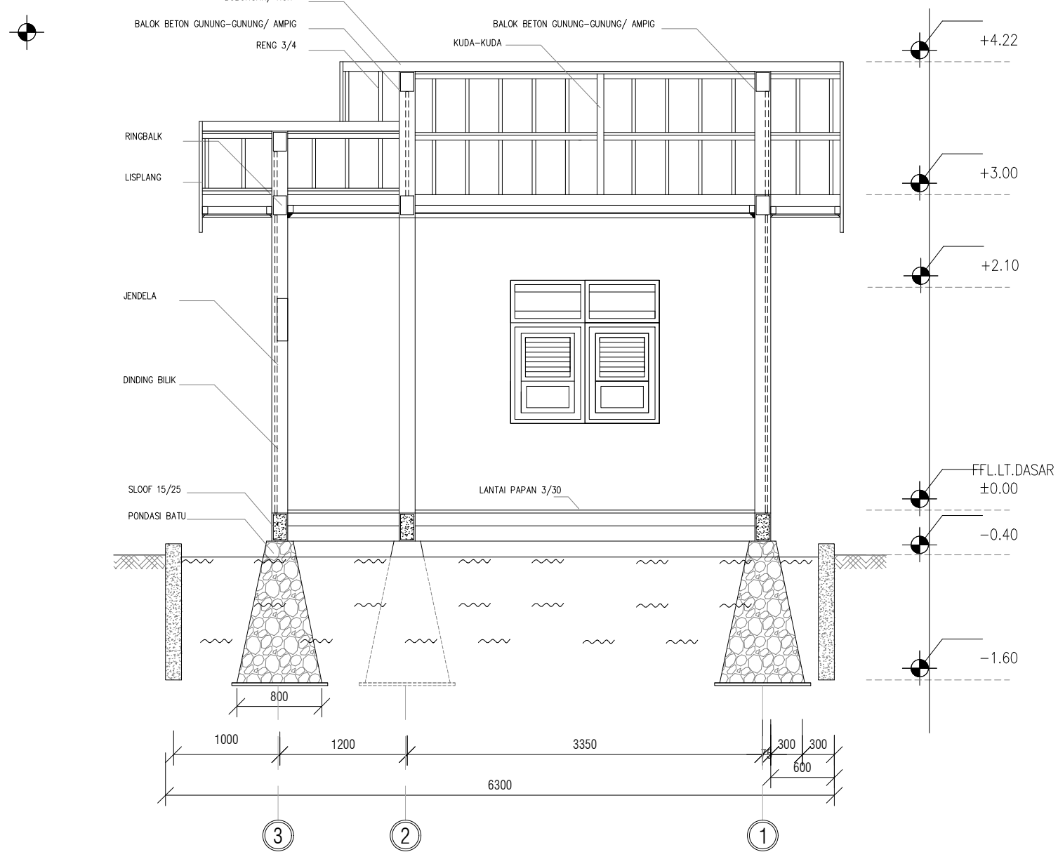
ARS POTONGAN B-B SKALA 1:50
