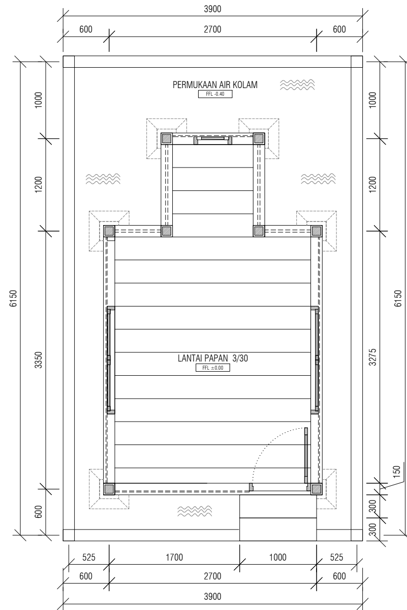
RENC. POLA LANTAI SKALA 1 : 50
