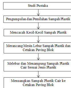
Gambar 2. Alur Kegiatan
