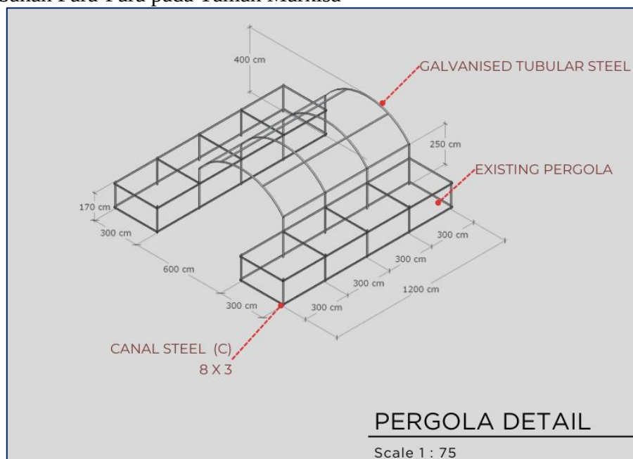
Gambar 19. Penambahan para-para disisi kanan dan pergola
