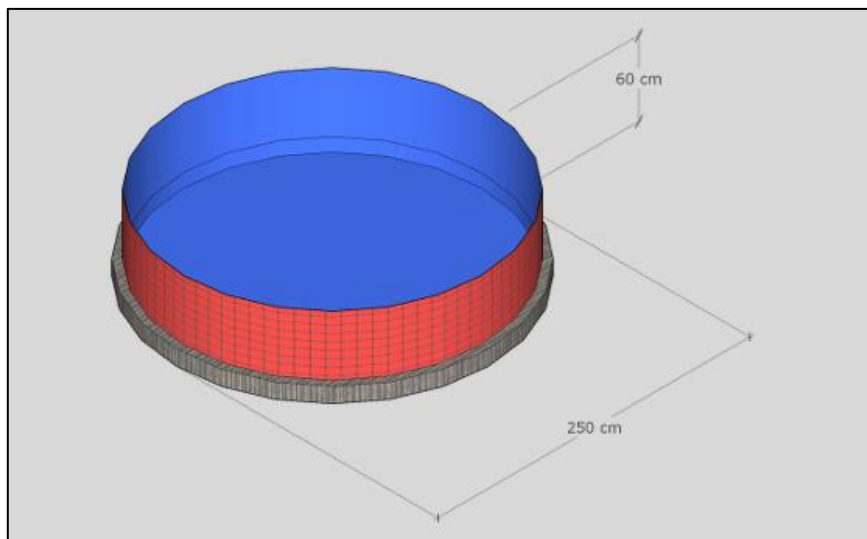
Gambar 21. Desain kolam biofloc budidaya ikan
