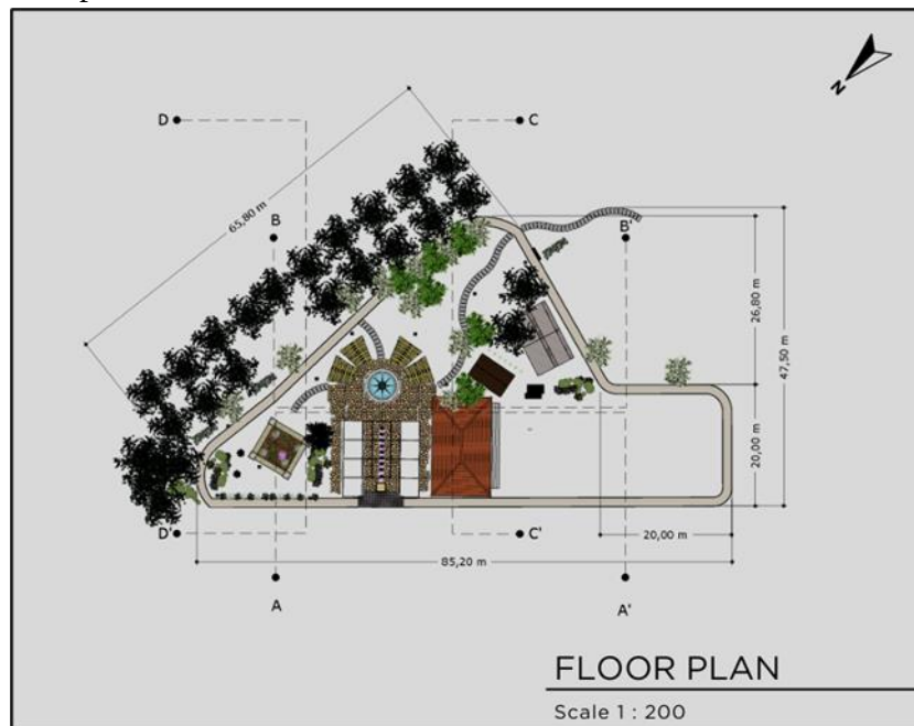
Gambar 6. Floorplan dan ukuran site yang direncanakan.
