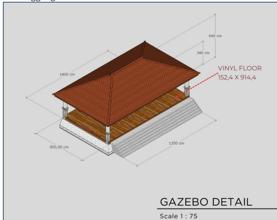
Gambar 18. Desain bangunan fungsi panggung
