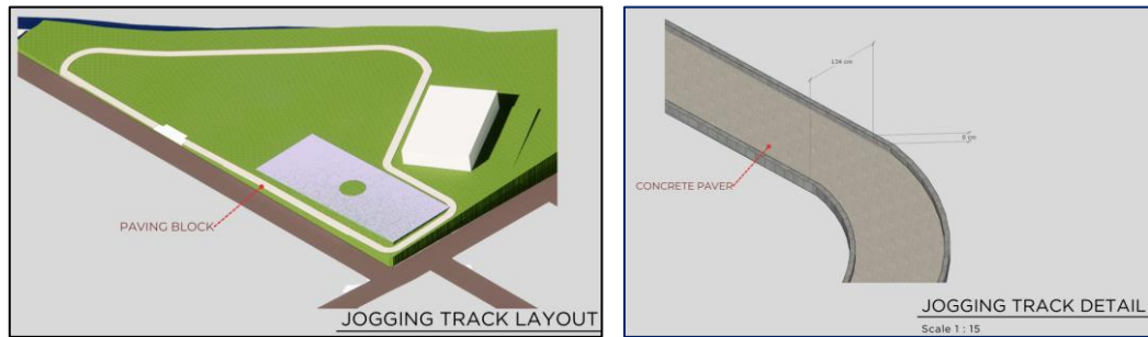
Gambar 20. Desain dan pola jogging track yang mengelilingi taman
