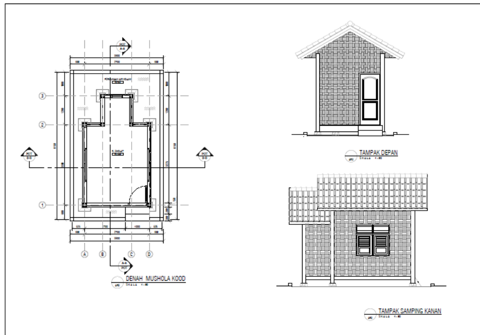
Gambar 3.3. Gambar DED untuk Mushollah di Kawasan rumah budaya
