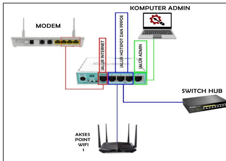
Gambar 7. Topologi Wi-Fi
