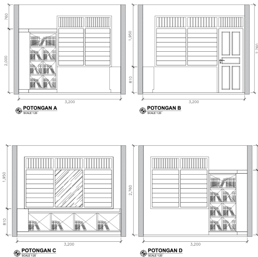
Gambar 3.7. Gambar Potongan
