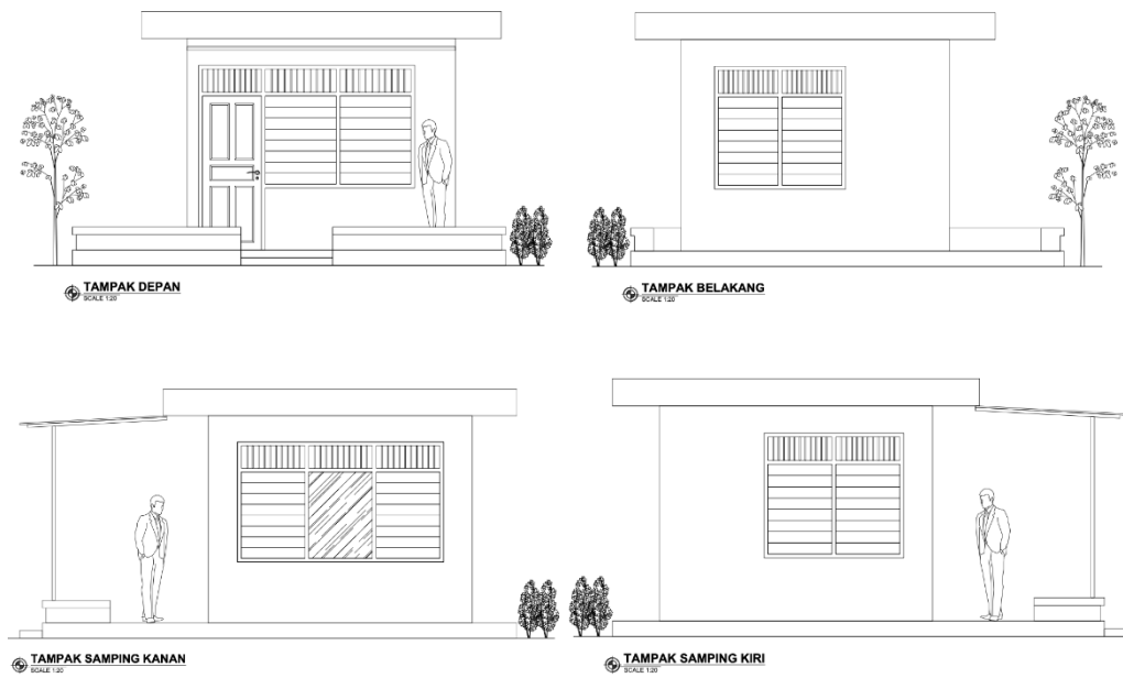
Gambar 3.6. Gambar Tampak
