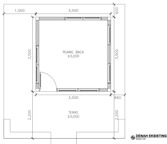
Gambar 3.5. Denah Pojok Baca
